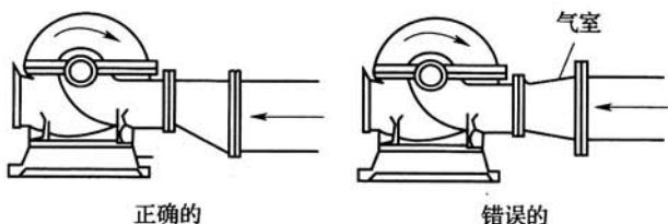
图4 正确和错误的水泵吸水管安装示意
