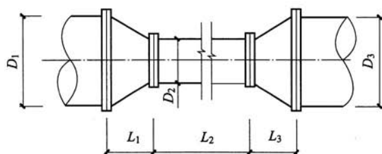
图 3 节流管结构示意图
