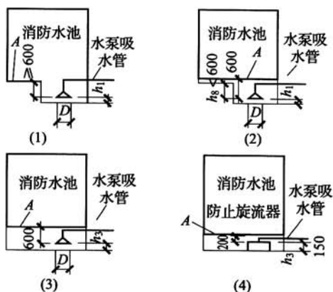
图2 消防水池最低水位
